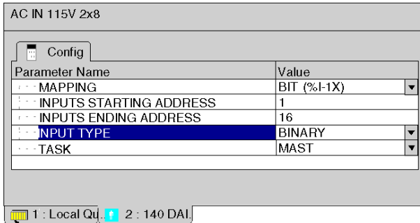
Parameter Configuration Window
