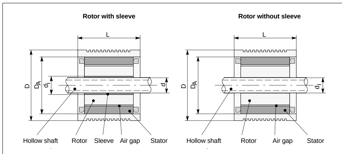
Fig. 1-3 Dimensions
