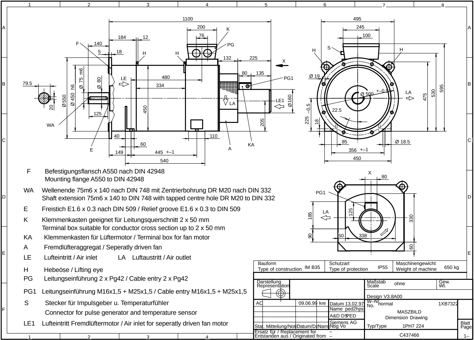
Fig. 4-28 1PH7 224, type of construction IM B35, air flow direction (DE → NDE)
