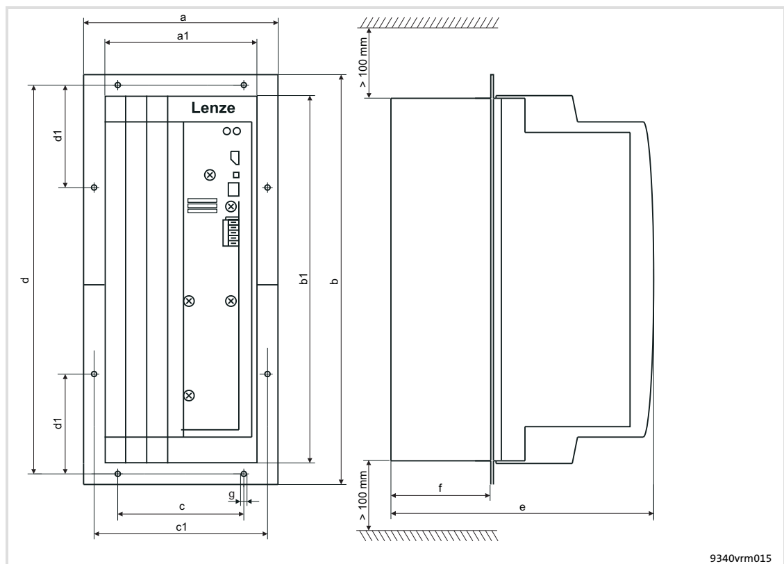
Fig.4-4 Encombresments des modules EMB9341-E et EMB9342-E en cas de montage traversant
